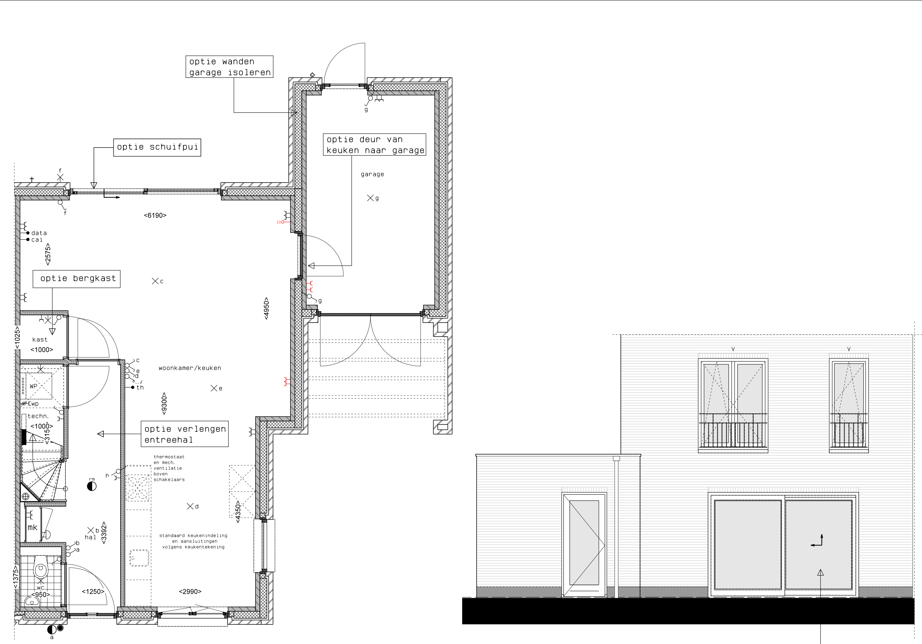
begane grond
