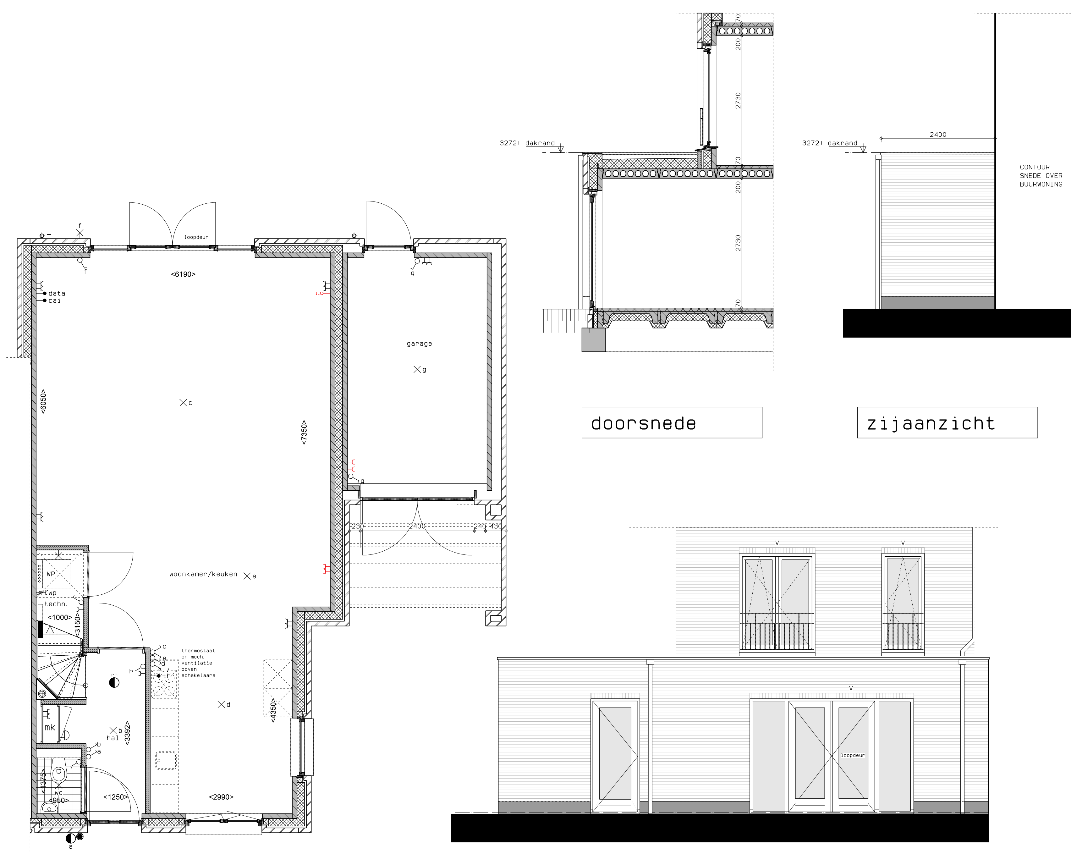
begane grond
