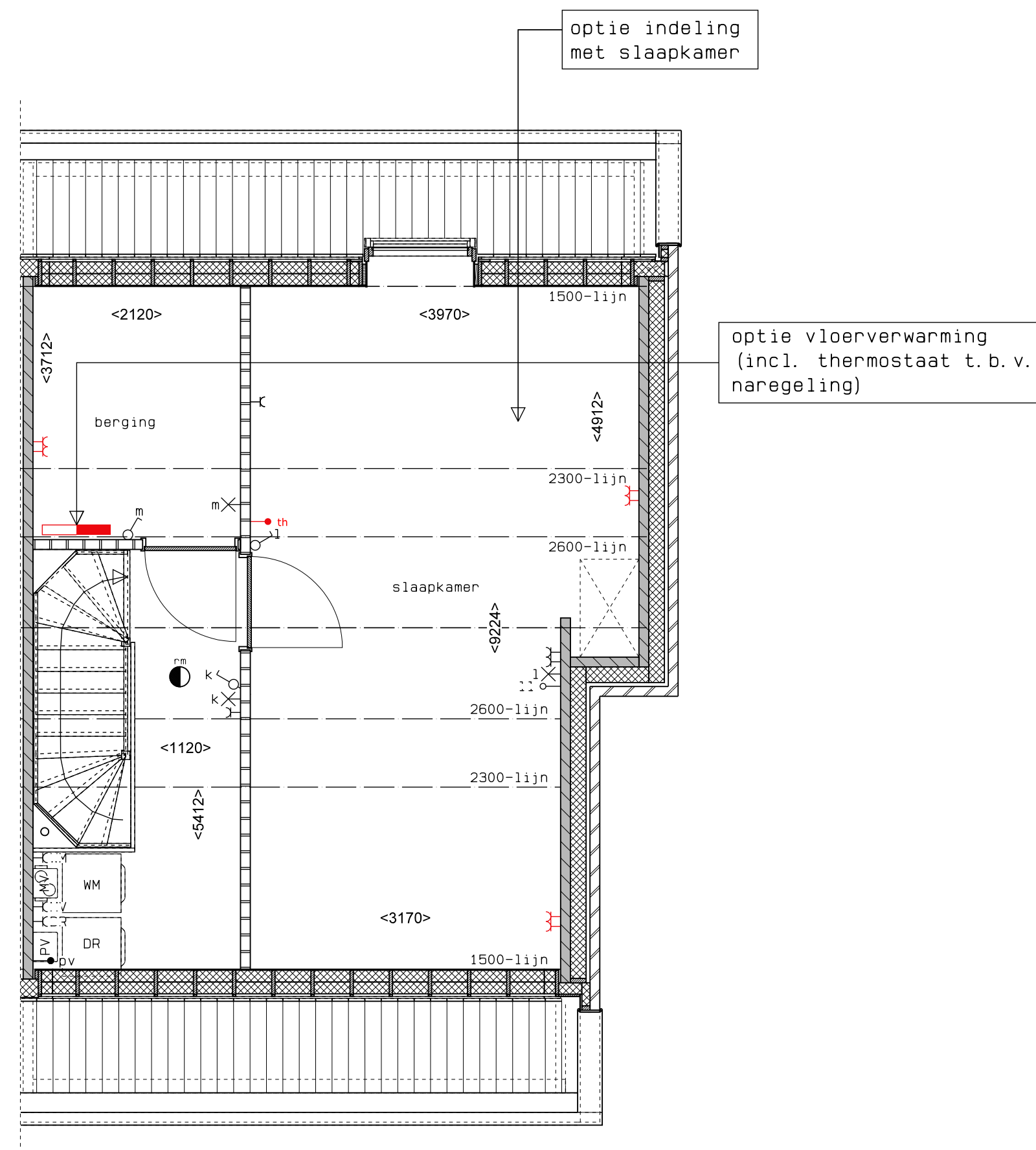
2e verdieping
